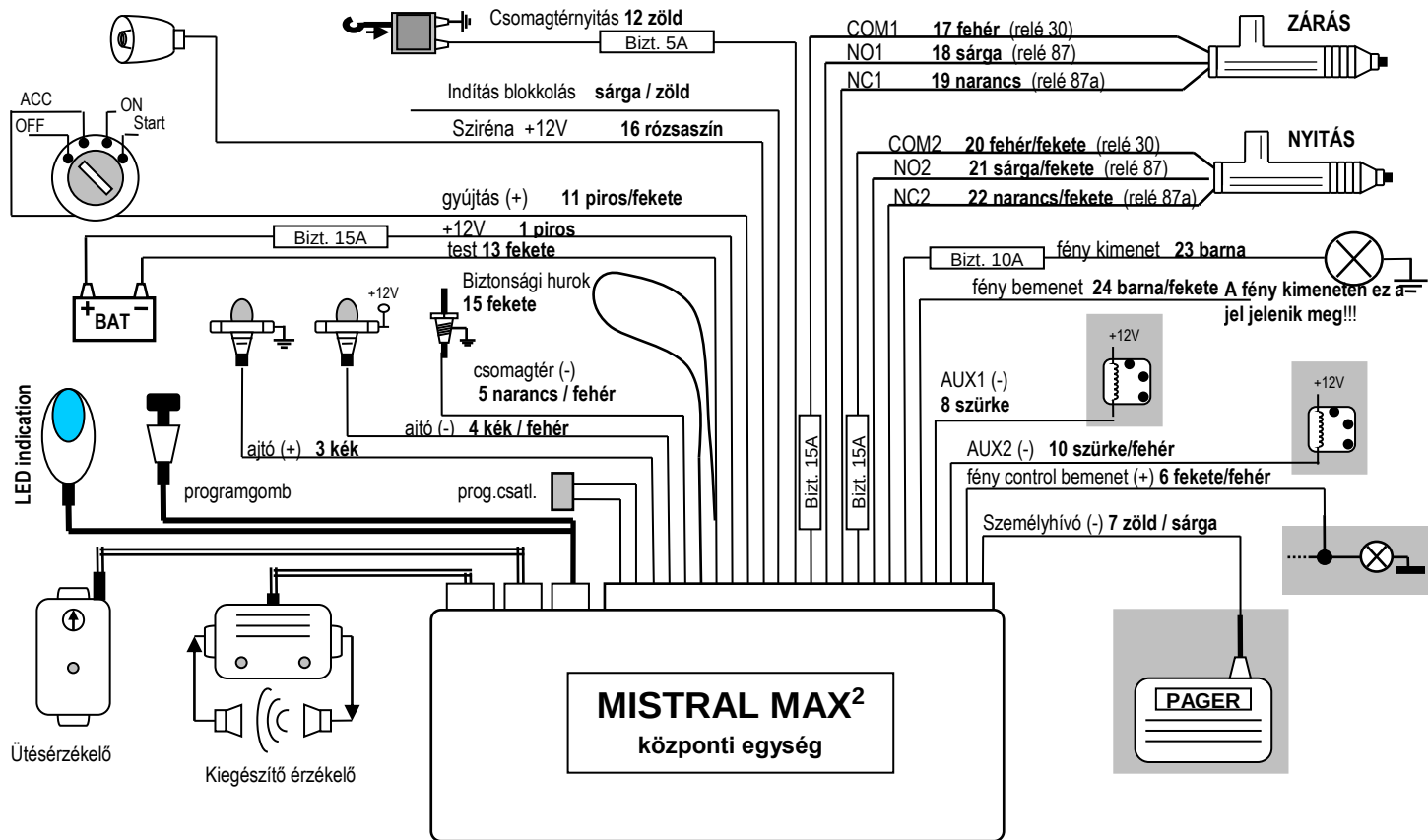
Riasztó bekötési rajz
