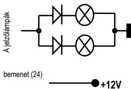
Jelzőlámpák bekötése példa
