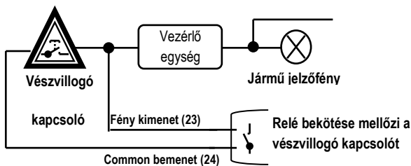
Parkoló fények kimenet a vészvillogóhoz kapcsolóhoz csatlakozik
