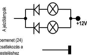
Parkoló fények kimenet a vészvillogóhoz kapcsolóhoz csatlakozik
