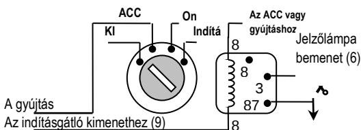
Az indításgátló kapcsolási rajza
